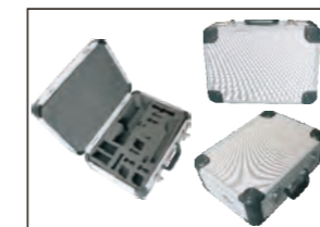
ITEM:APC018 Material:AL,ABS I D:L450×W320×H145 mm OD:L460×W330×H155 mm
